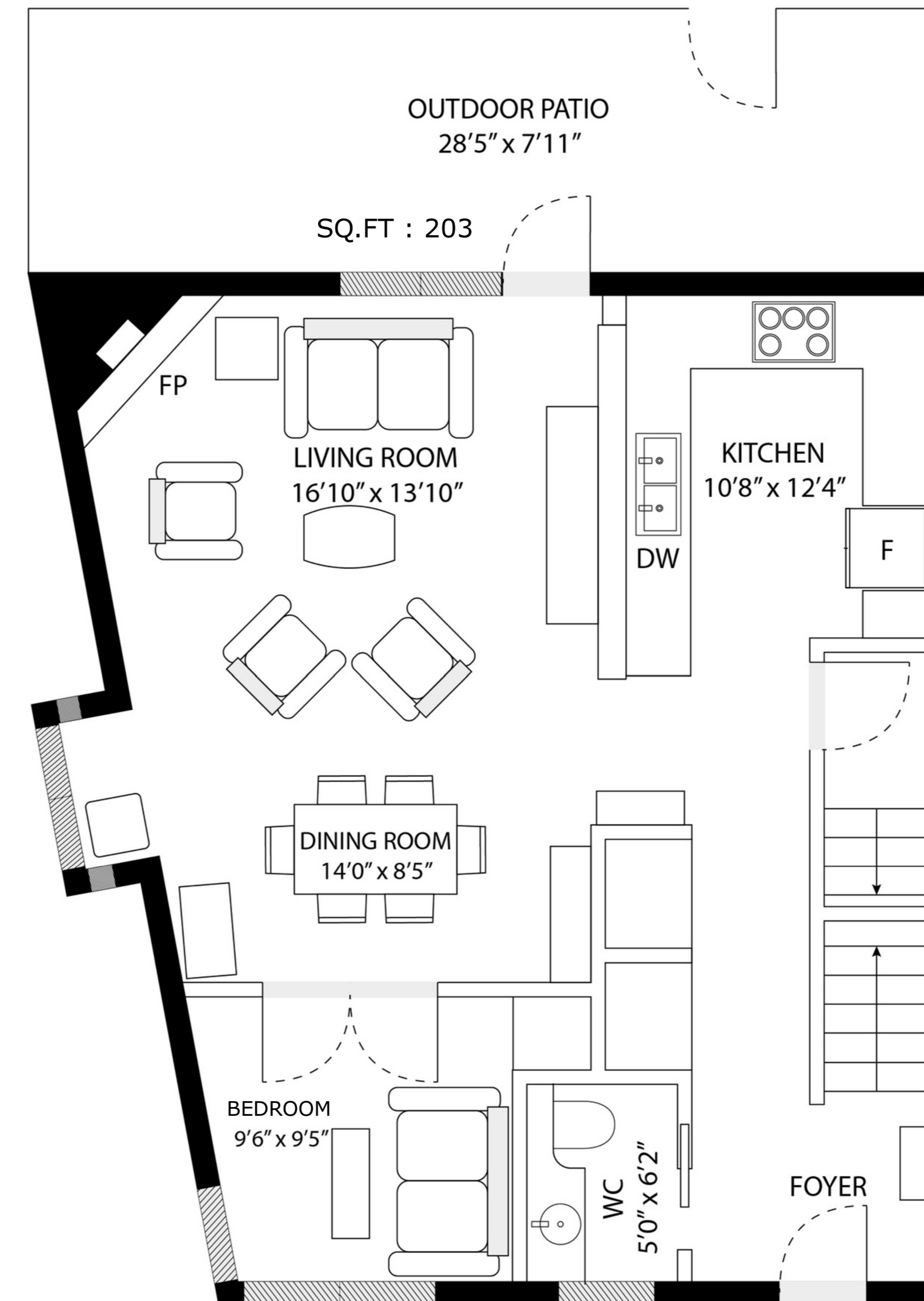
MAIN FLOOR SQ.FT : 841
